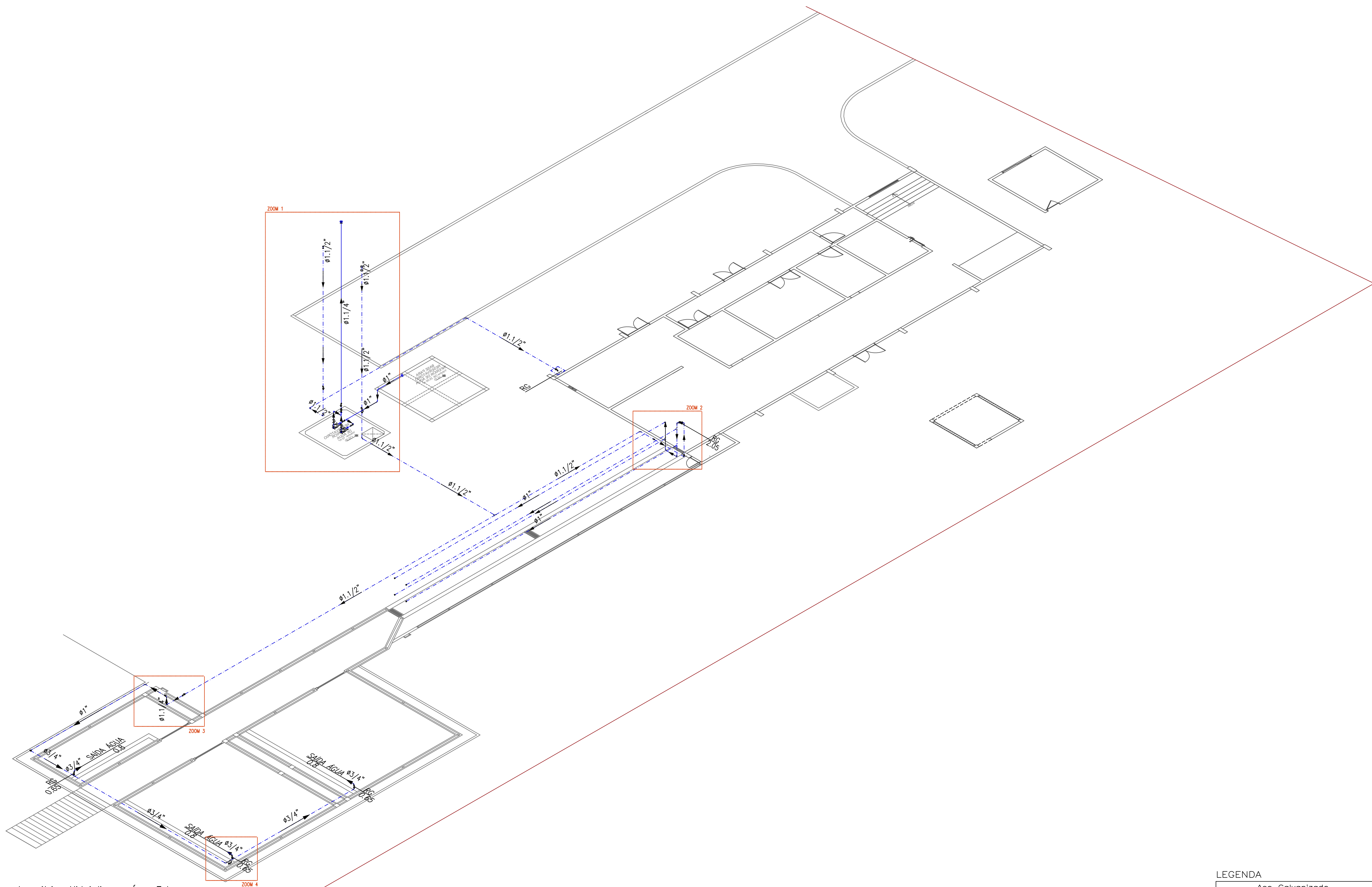
Isométrico Hidráulico – Área Externa
